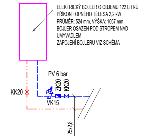
SCHEMA ZAPOJENÍ EL. BOJLERU:
